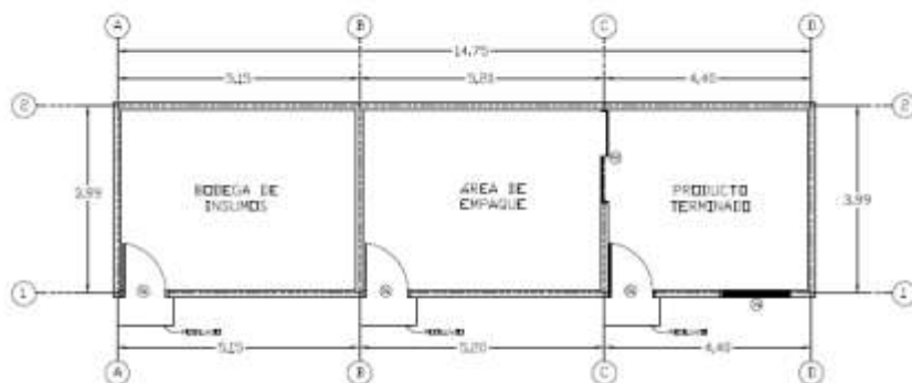
PLANTA CONSTRUCTIVA
