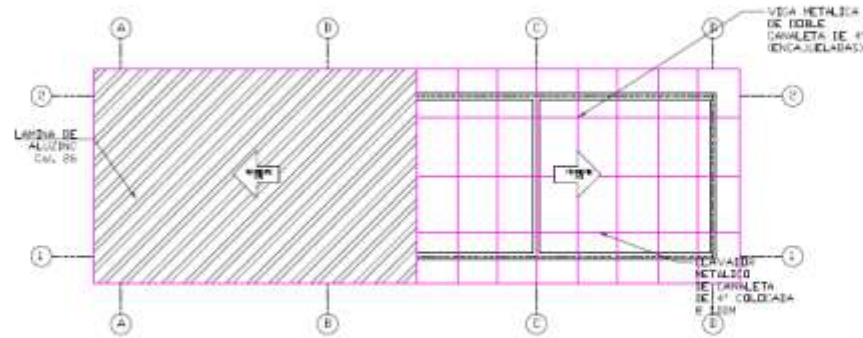
PLANTA ESTRUCTURAL DE TECHO
