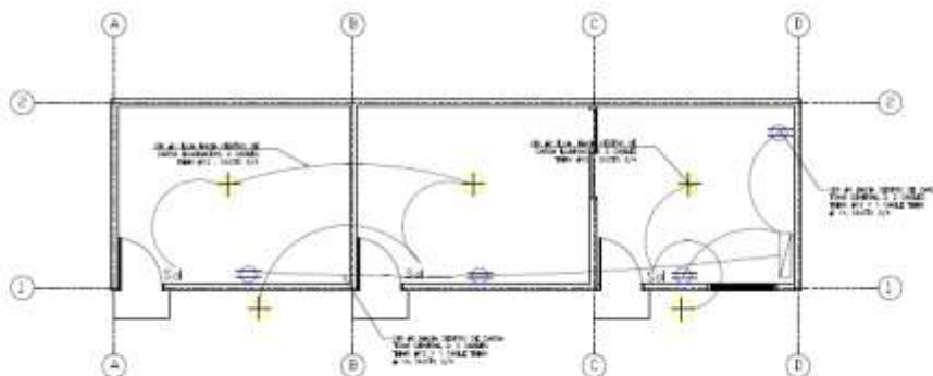
PLANTA DE INSTALACIONES ELÉCTRICAS
