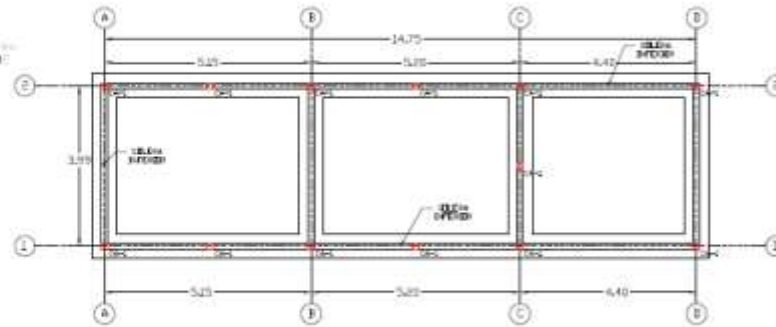
PLANTA DE CIMENTACIÓN
