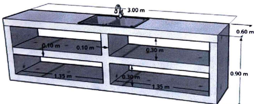
DETALLE MUEBLE DE COCINA
